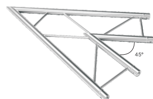
RKLA22H-21 45° 2WAY CH-21
