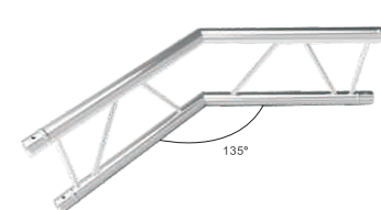
RKLA22V-25 135° 2WAY CV-25
