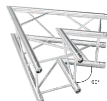
RKSQ12-22 60° 2WAY C-22
