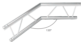
RKLA29V-25 135° 2WAY CV-25
